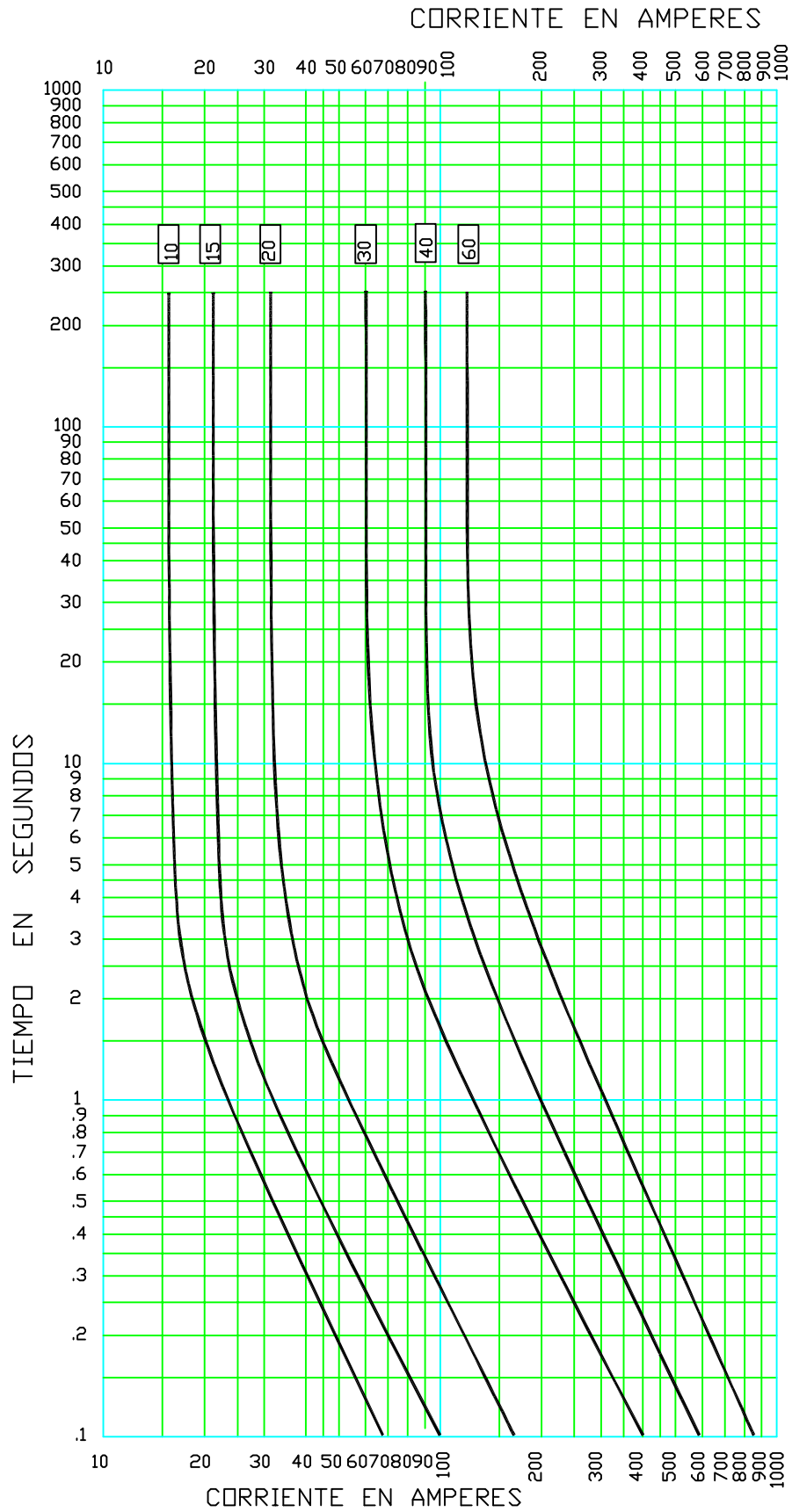
CURVAS CARACTERÍSTICAS CORRIENTE - TIEMPO DE FUSIÓN Alambre Calibrado Capacidades Preferidas Tolerancia +/-20%.
